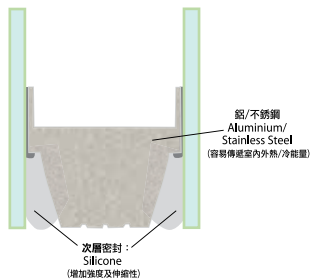
高分子發泡隔條
