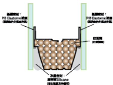
不銹鋼加絕緣塗層隔條
